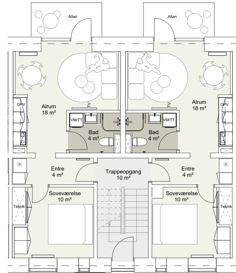
GL. LANDEVEJ 162 ST.TV. BBR-AREAL : 51 m² ANTAL VÆRELSE : 2 værelse
