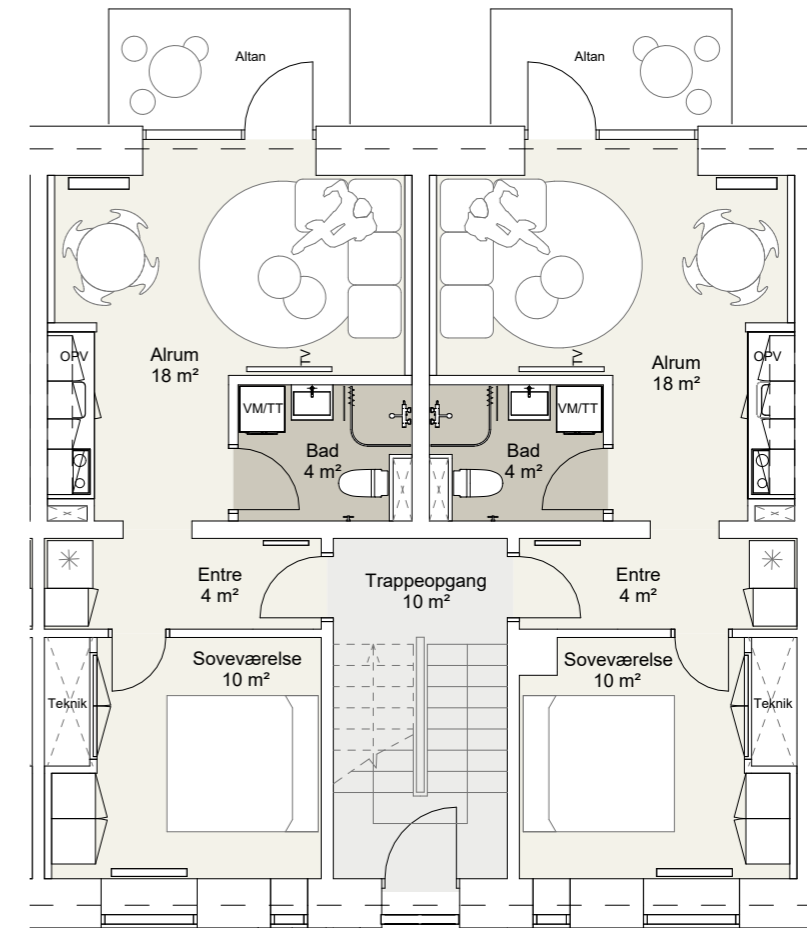
LANDEVEJ 166 ST.TV. BBR-AREAL : 50 m² ANTAL VÆRELSE : 2 værelse
