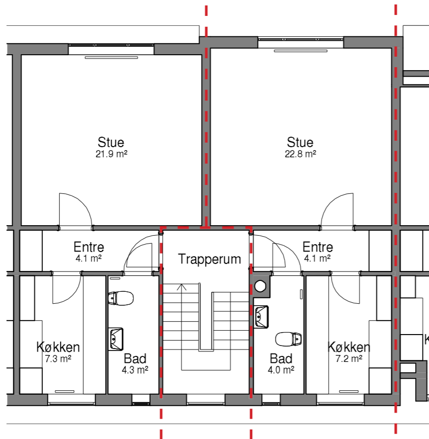
LANDEVEJ 166 2.TV. BBR-AREAL : 48,8 m² TYPE : K-1-1V ANTAL VÆRELSE : 1 værelse
