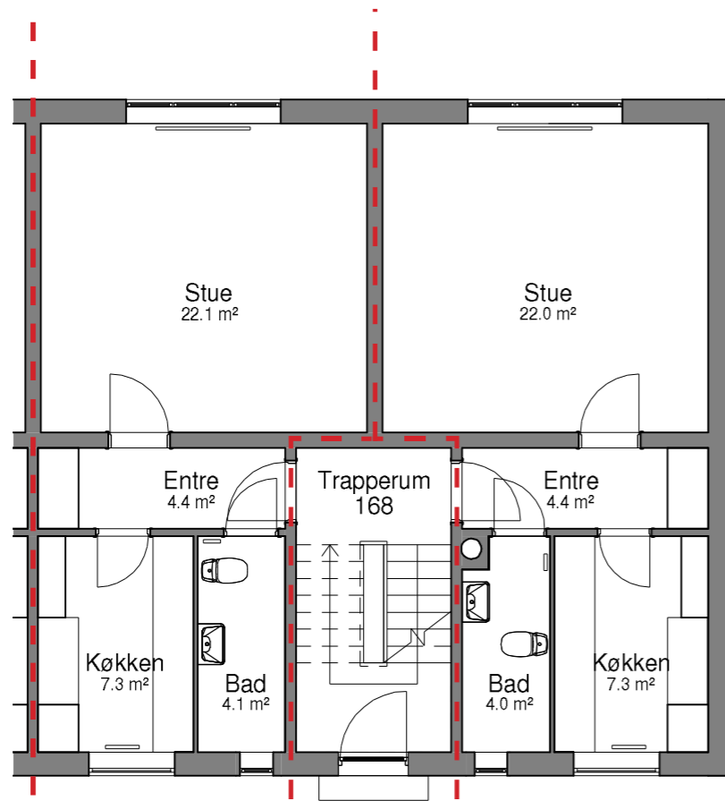
LANDEVEJ 168 ST.TV. BBR-AREAL : 51,1 m 2 TYPE : K-1-1V ANTAL VÆRELSE : 1 værelse
