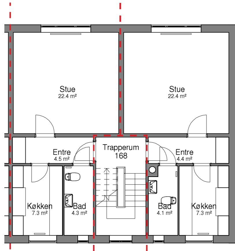
LANDEVEJ 168 1.TV. BBR-AREAL : 51,1 m 2 TYPE : K-1-1V ANTAL VÆRELSE : 1 værelse
