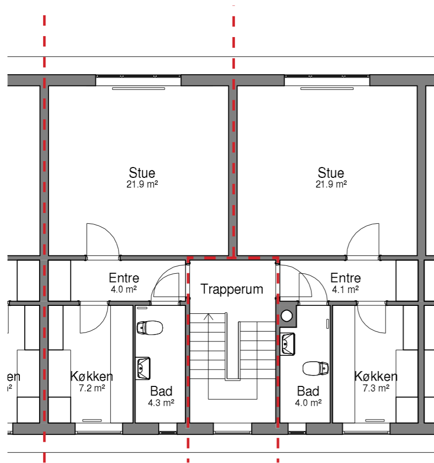
GL. LANDEVEJ 164 2.TV. BBR-AREAL : 48,8 m 2 TYPE : K-1-1V ANTAL VÆRELSE : 1 værelse
