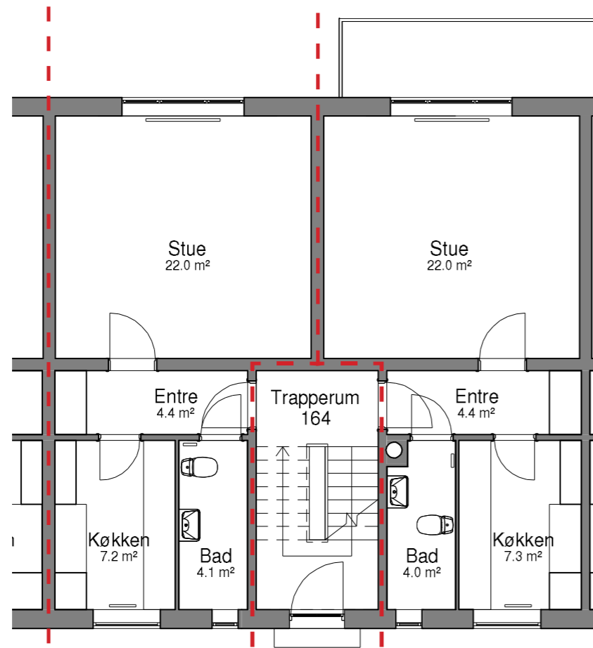
GL. LANDEVEJ 164 ST.TV. BBR-AREAL : 50,5 m² TYPE : K-1-1V ANTAL VÆRELSE : 1 værelse
