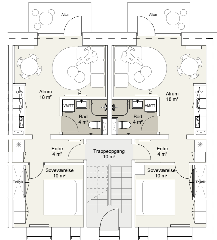
LANDEVEJ 168 ST.TV. BBR-AREAL : 51 m 2 ANTAL VÆRELSE : 2 værelse
