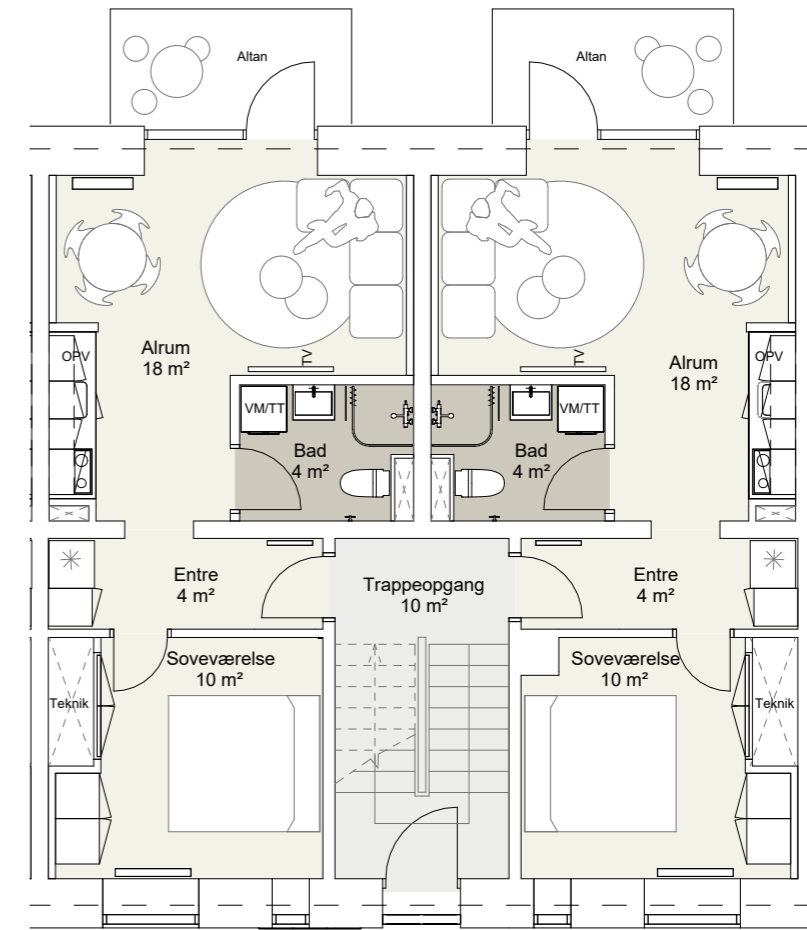
GL. LANDEVEJ 164 ST.TV. BBR-AREAL : 51 m² ANTAL VÆRELSE : 2 værelse
