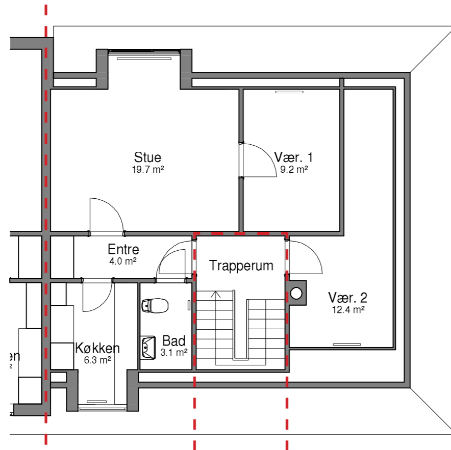
LANDEVEJ 168 2. BBR-AREAL : 71,2 m² TYPE : K-2-3V ANTAL VÆRELSE : 3 værelser
