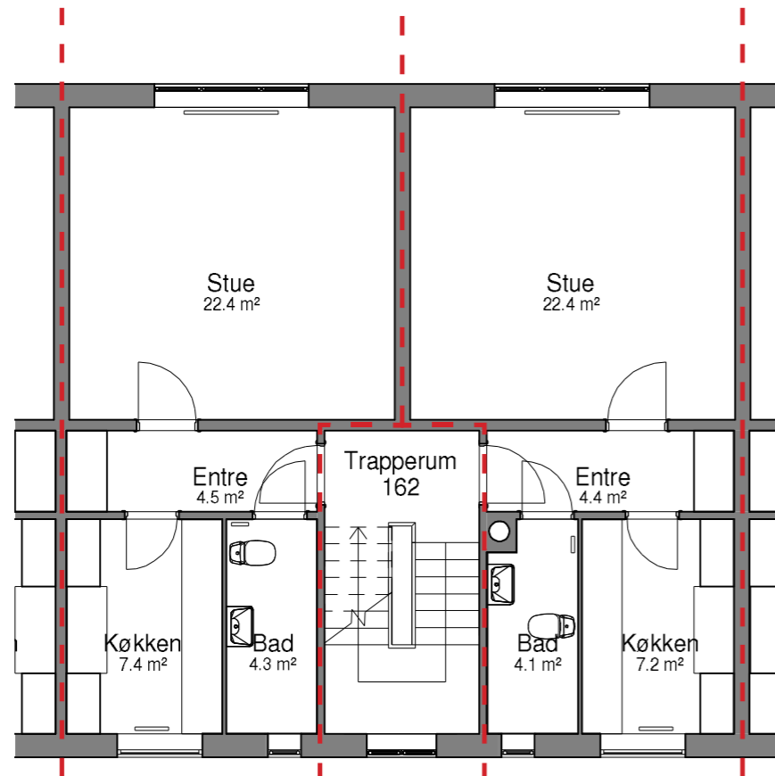
GL. LANDEVEJ 162 1.TV. BBR-AREAL : 50,4 m² TYPE : K-1-1V ANTAL VÆRELSE : 1 værelse
