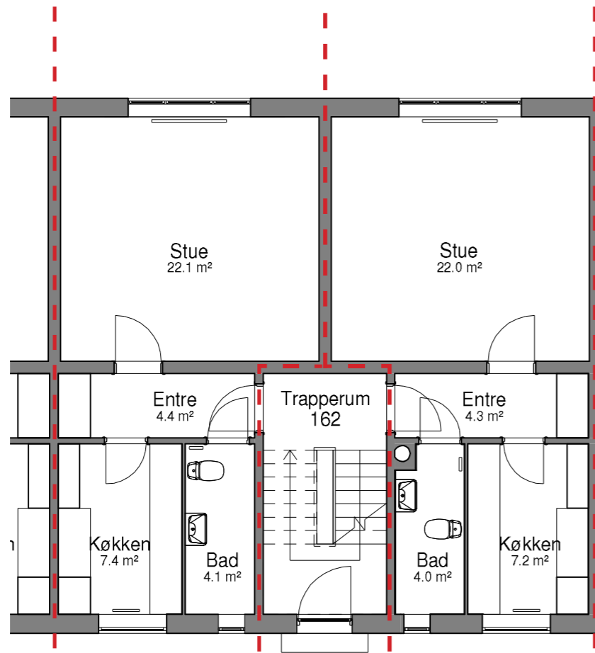
GL. LANDEVEJ 162 ST.TV. BBR-AREAL : 50,4 m² TYPE : K-1-1V ANTAL VÆRELSE : 1 værelse
