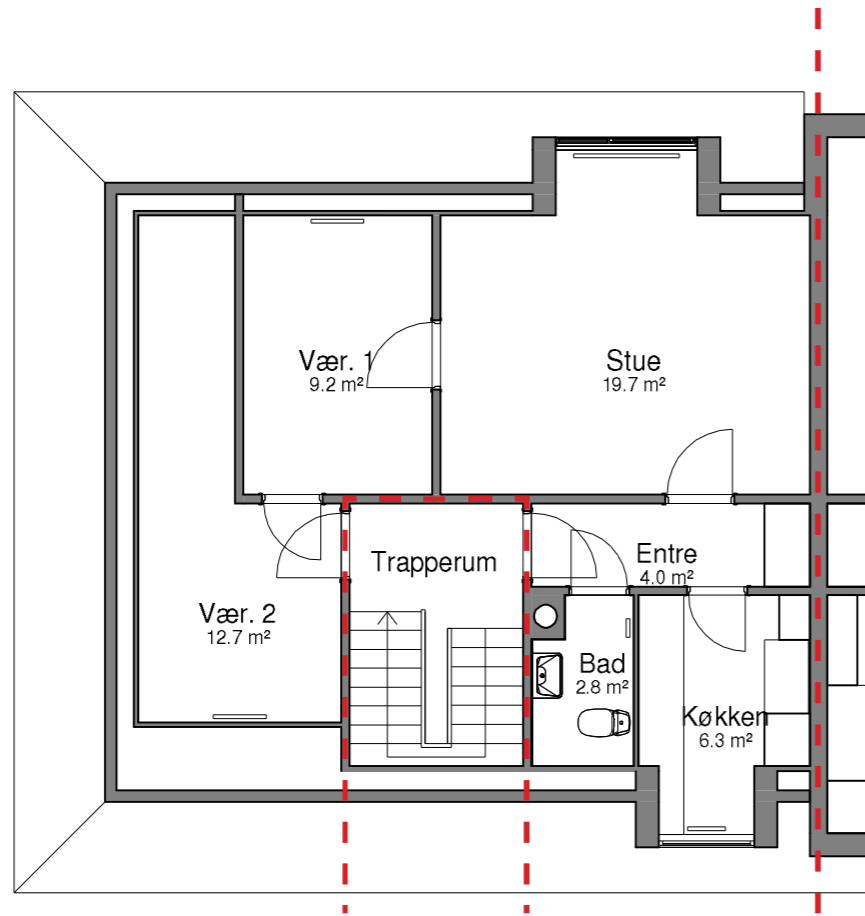
GL. LANDEVEJ 160 2. BBR-AREAL : 71,2 m² TYPE : K-2-3V ANTAL VÆRELSE : 3 værelser
